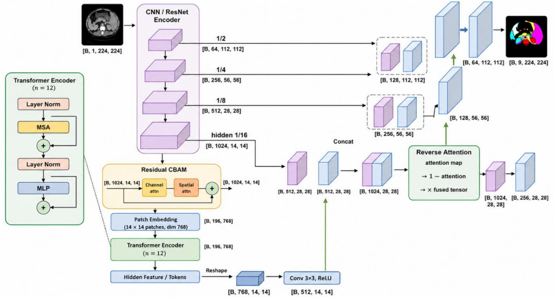
Hình 3.6. Reverse Attention sau phép nối decoder-skip đầu tiên.
