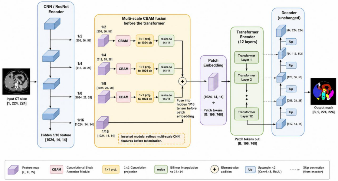
Hình 3.4. Vị trí khảo sát CBAM đa tỷ lệ trong pipeline TransUNet.
