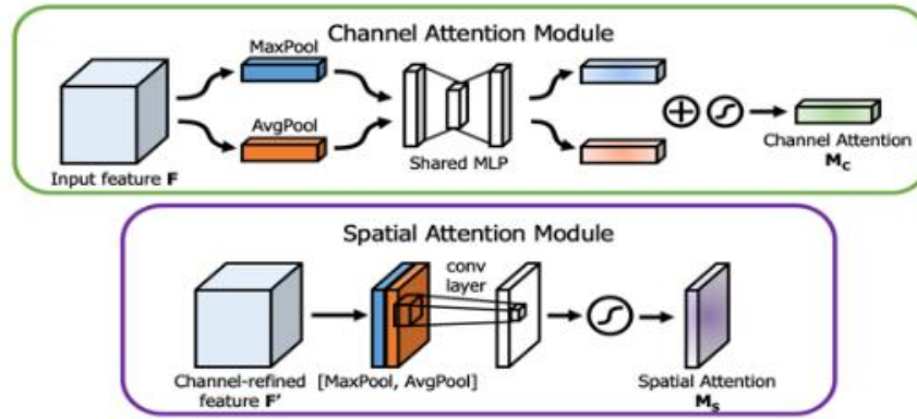
Hình 2.1. Sơ đồ chi tiết hai mô-đun chủ yếu thành phần của CBAM [9].
