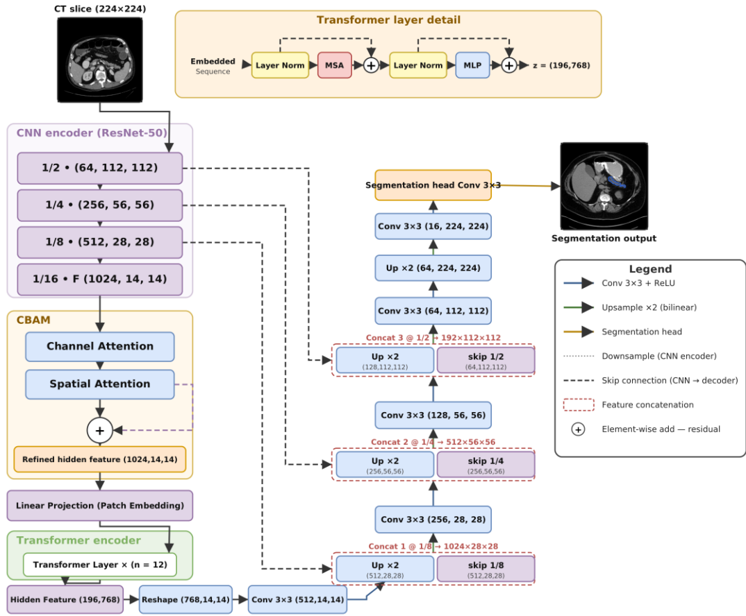
Hình 3.3. Kiến trúc CBAM-TransUNet đề xuất: khối CBAM phân dư tính chỉnh bản đồ đặc trưng CNN ở tỷ lệ 1/16 ngay trước bước tạo token; bộ mã hóa Transformer và bộ giải mã giữ nguyên như cấu hình nền.
